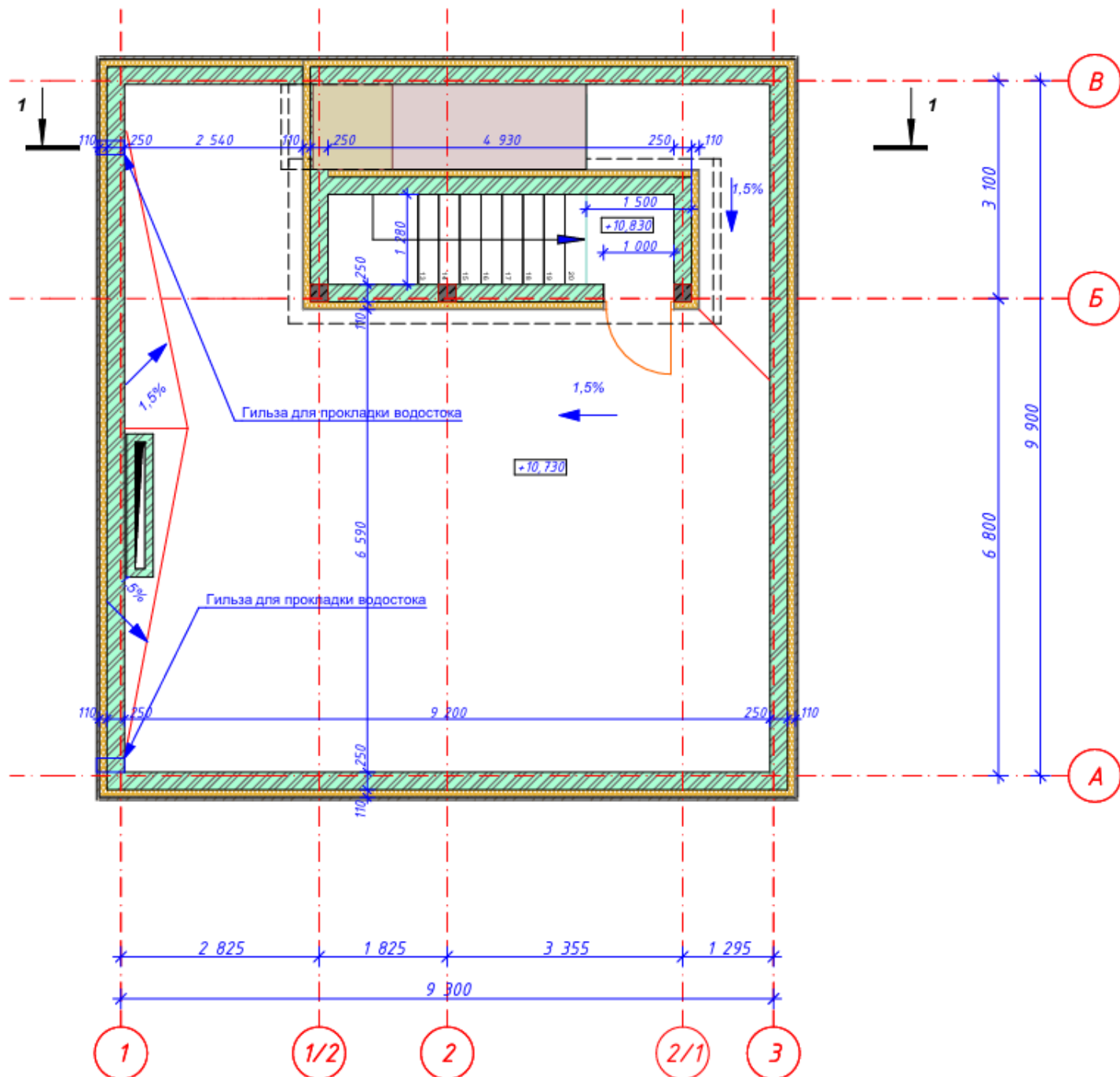
Илл.9. План кровли
