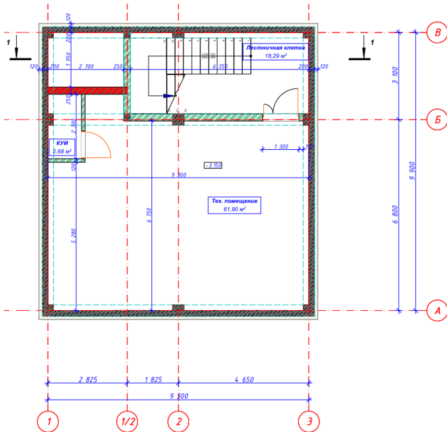
Илл.5. План подвального этажа на отм. -3,150
