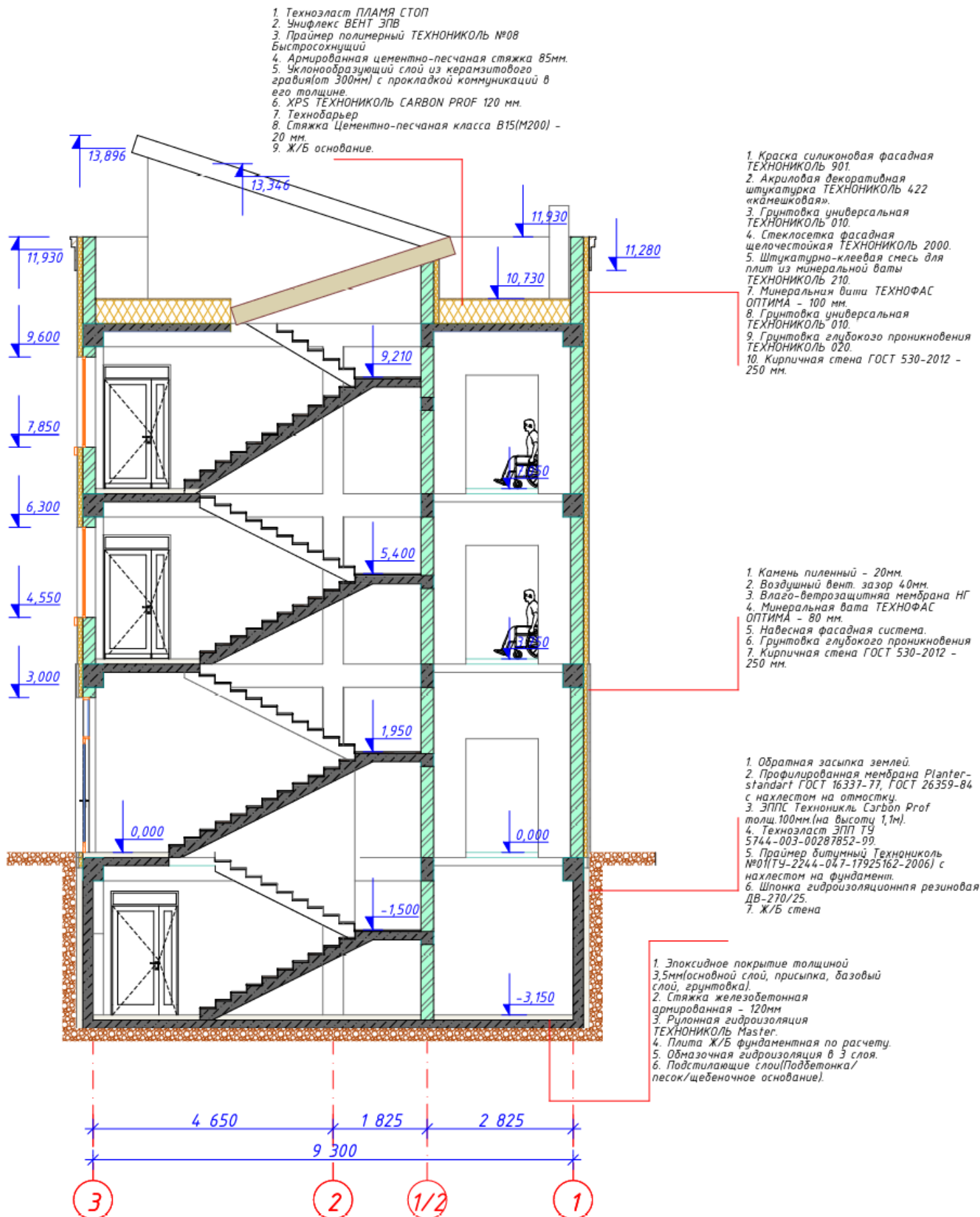
Илл. 10. Разрез I-I
