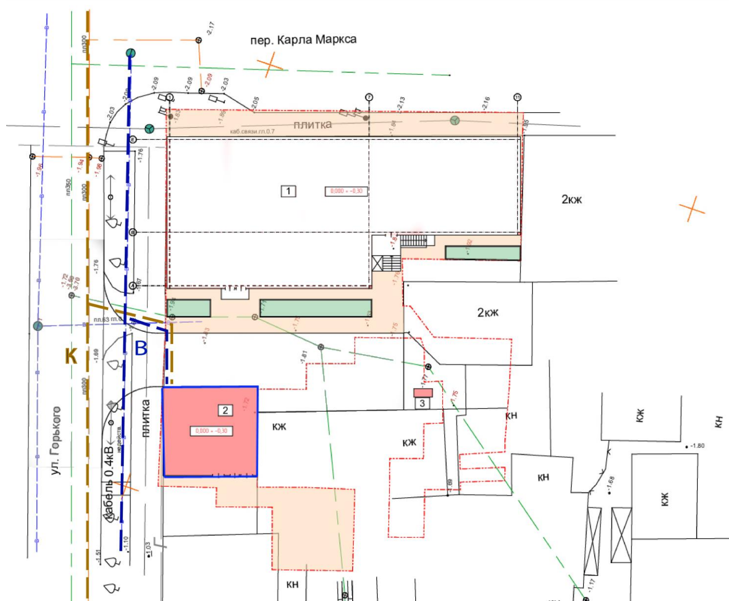
Рис. 1. Сводный план инженерных сетей
