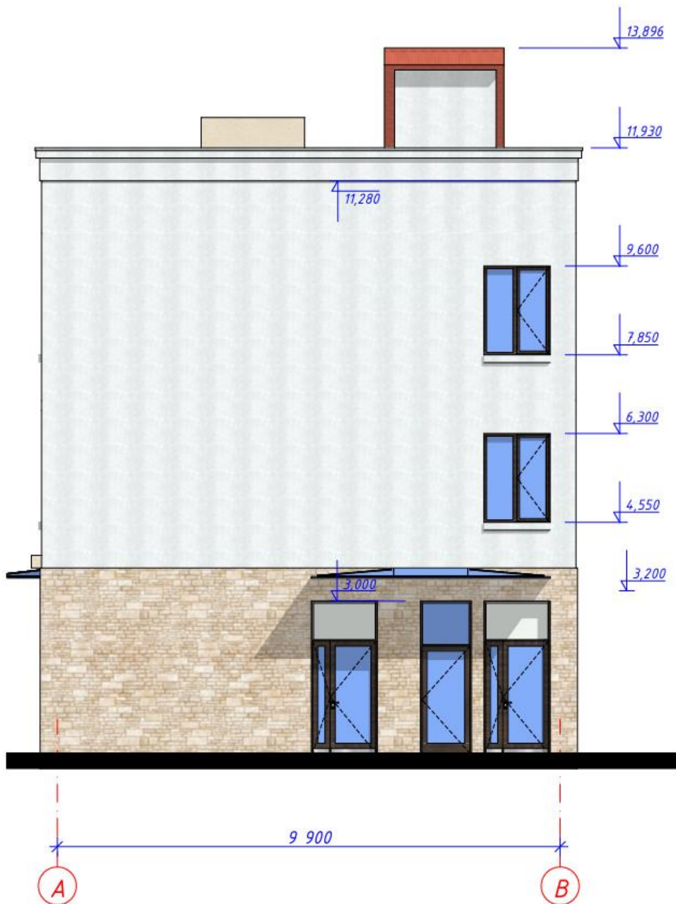
Илл. 13. Фасад в осях А-В
