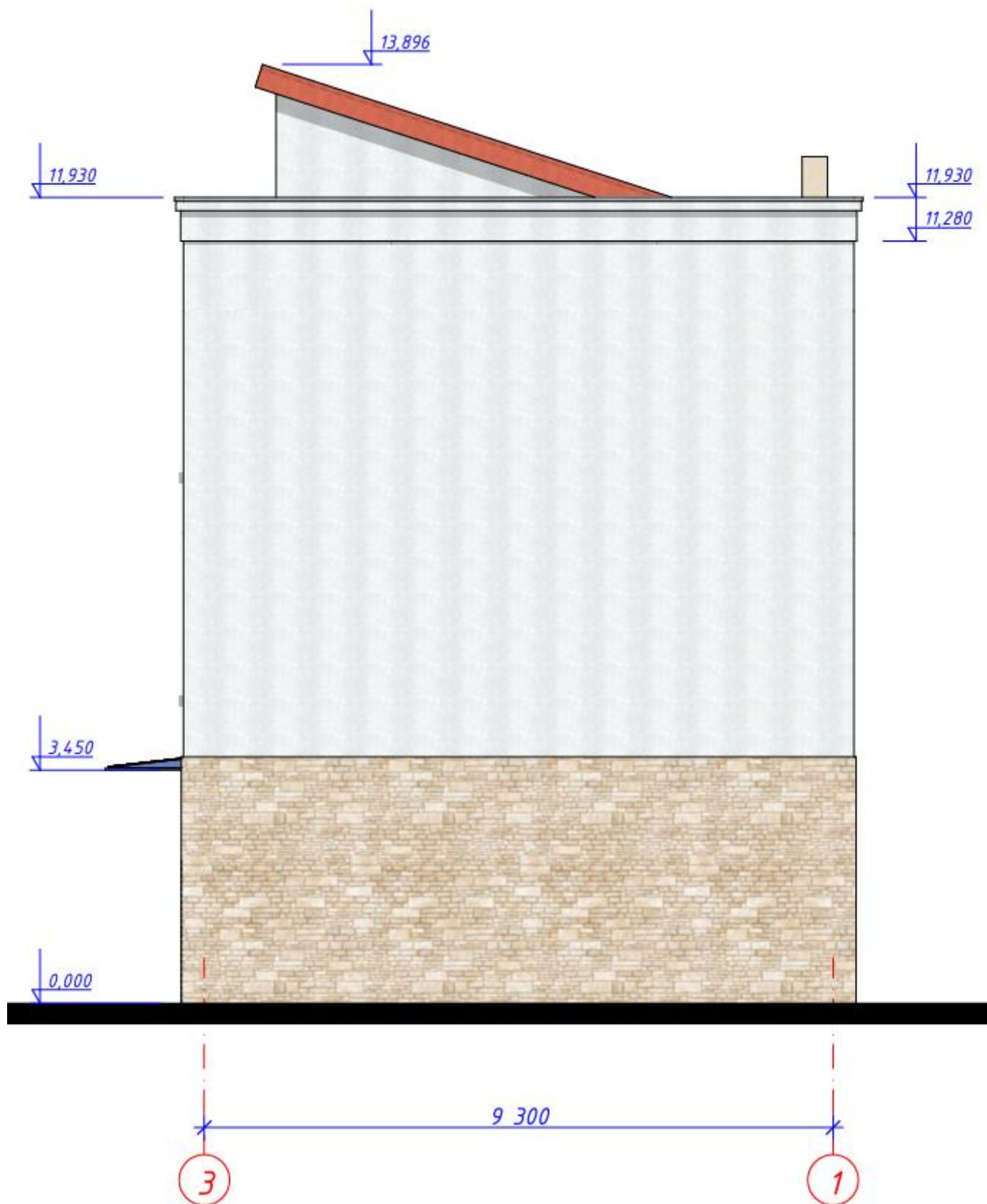
Илл. 12. Фасад в осях 3-1
