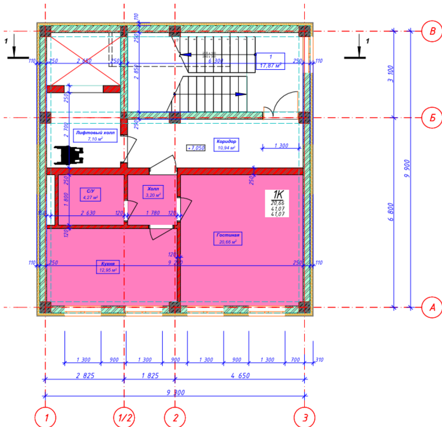
Илл.8. План третьего этажа
