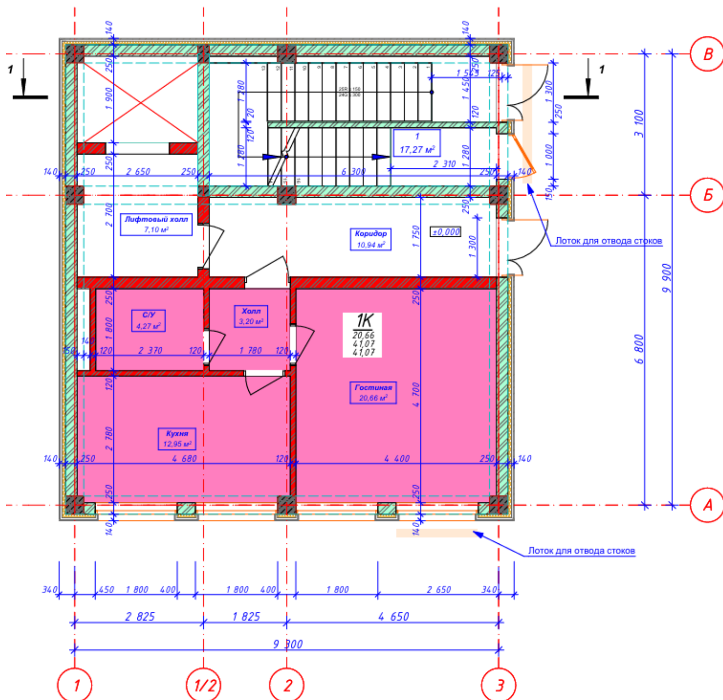
Илл.6. План первого этажа на отм. 0,000
