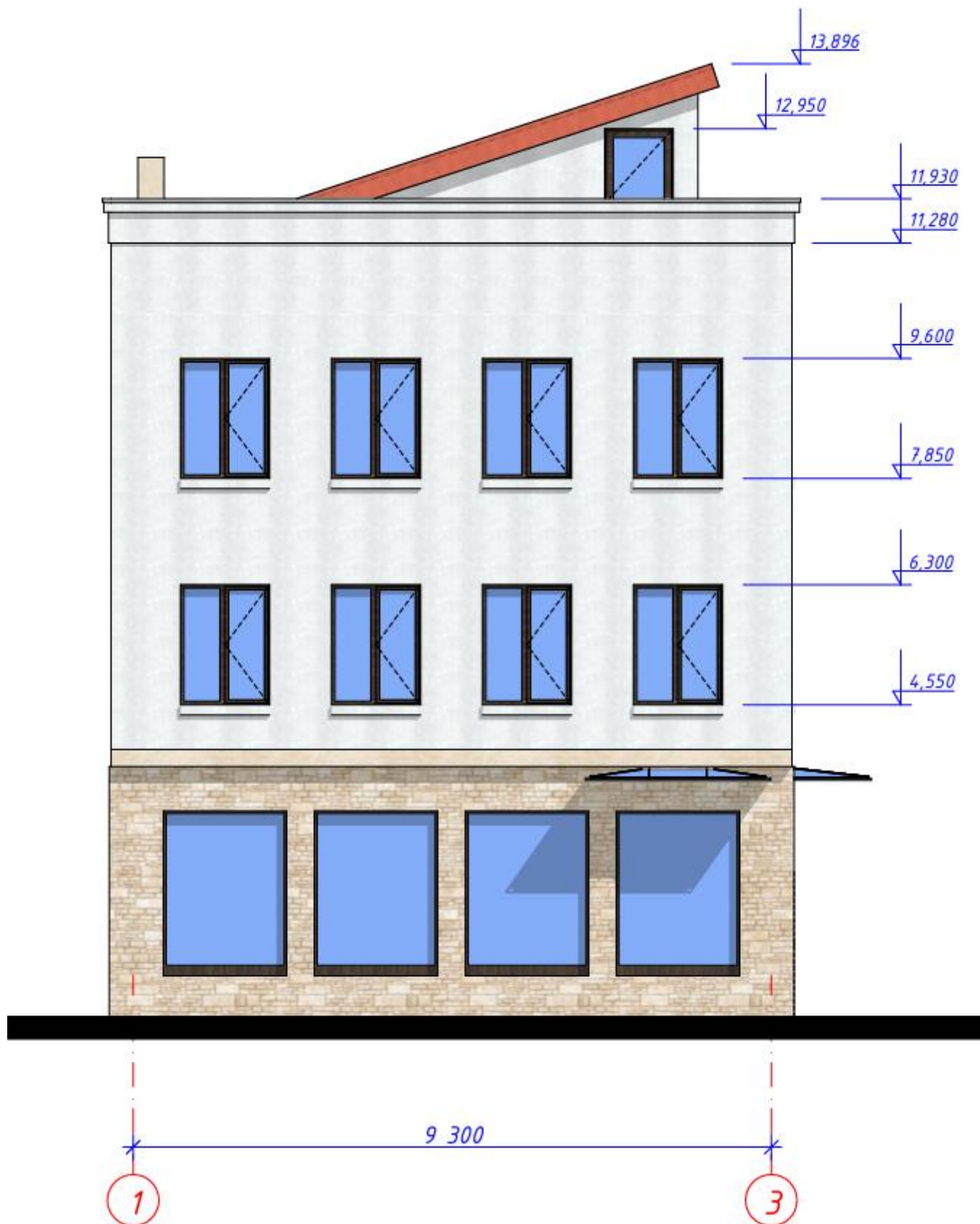
Илл. 11. Фасад в осях I-3
